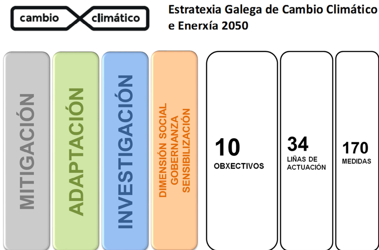
[Figura 4].- Esquema de definición de obxectivos, liñas de actuación e medidas da Estrutura da Estratexia Galega de Cambio Climático e Enerxía 2050 . Fonte: Elaboración propia
