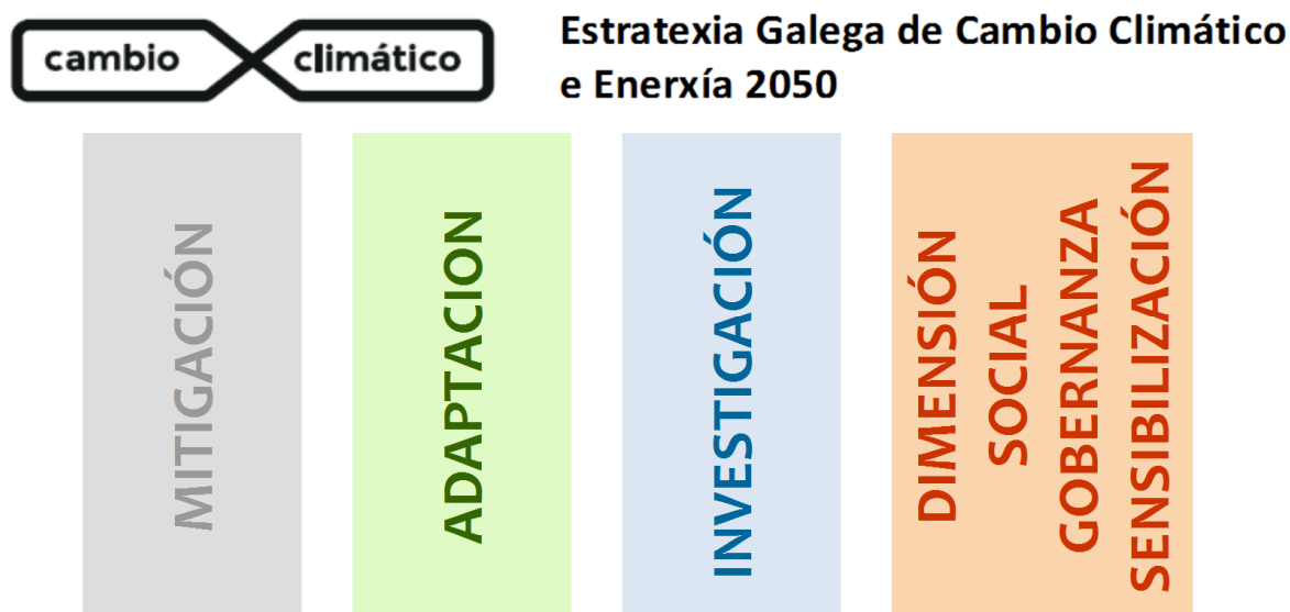
[Figura 1].- Ámbitos de actuación da Estratexia Galega de Cambio Climático e Enerxía 2050 Fonte: Elaboración propia
