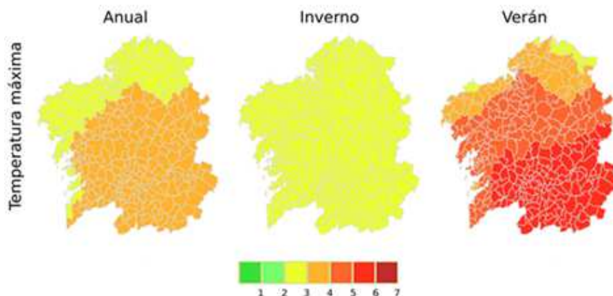
[Figura 19].- Cambio da temperatura máxima anual, en inverno e en verán en °C. Móstranse as diferenzas do valor medio 2061-2090 con respecto a 1971-2000 en °C. Para cada concello móstrase a mediana (el valor mais probable), das 11 proxeccións obtidas dos 11 modelos rexionais.
