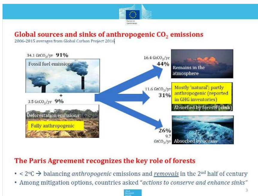
[Figura 14].- Fontes y sumidoiros de CO 2 Fonte: Comisión Europea
